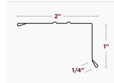
1"x2" STYLE A ROOF EDGE
