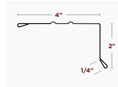
2"x4" STYLE A ROOF EDGE
