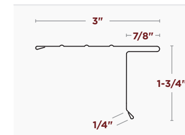
6" STYLE L ROOF EDGE
