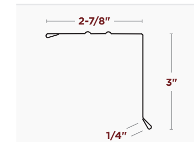
3"x3" STYLE A ROOF EDGE
