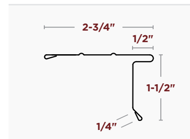
5" STYLE SR ROOF EDGE
