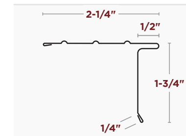
5" STYLE SRLL ROOF EDGE
