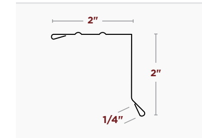
2"x2" STYLE A ROOF EDGE
